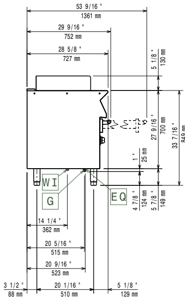
Zij aanzicht
